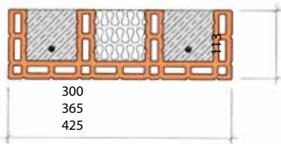
Lochbild 3) Wärmedämm-Ziegelsturz
